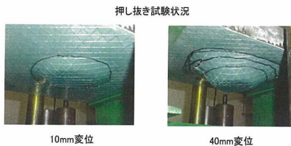
押し抜き試験結果
