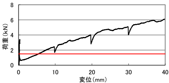
押し抜き試験
