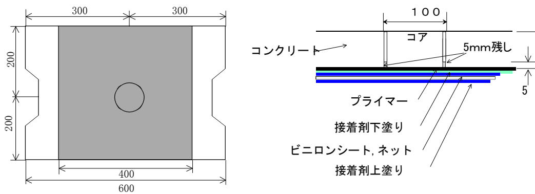
供試体概略図
